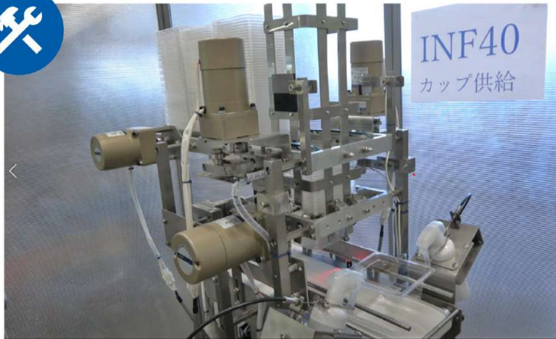
カップ供給装置
