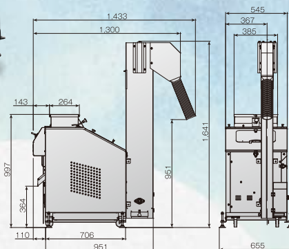
粉すり機
